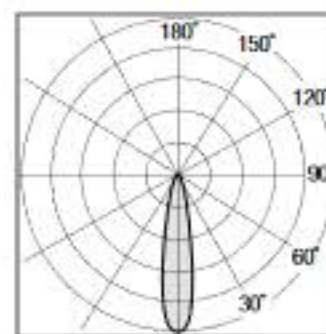
Diagramma Polare (12°)
