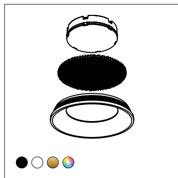
Ottica+Anello riflettore+honeycomb
