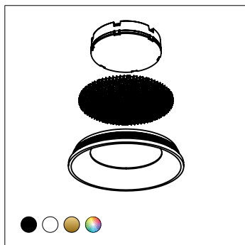
Ottica+Anello riflettore+honeycomb
